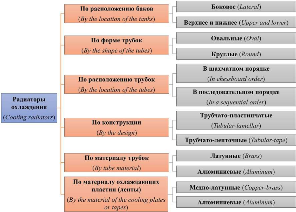
Рис. 3. Классификация радиаторов системы охлаждения ДВС Fig. 3. Classification of radiators of the cooling system of internal combustion engines
