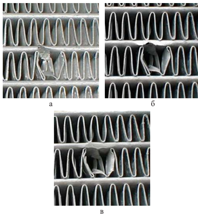
Рис. 5. Герметизация течи жидкости в радиаторе: а – дефект; б – подготовленная поверхность; в – восстановленная поверхность
