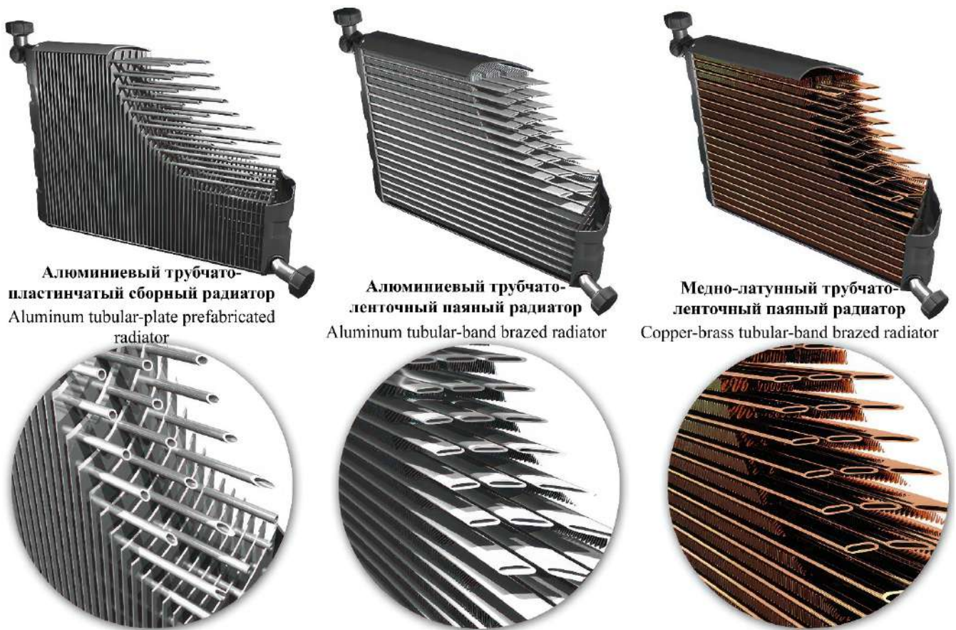
Рис. 2. Радиаторы, используемые в автотракторной технике Fig.2. Examples of radiators used in auto-tractor equipment
