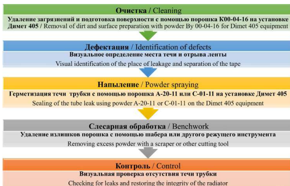
Рис. 6. Схема технологического процесса восстановления радиатора
